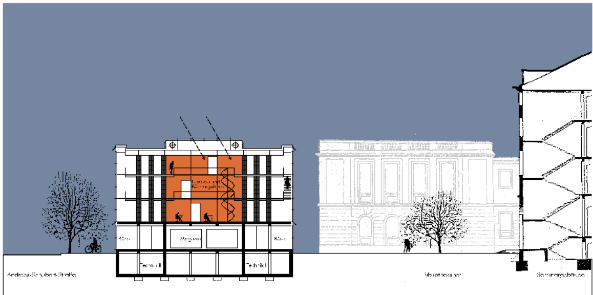
Querschnitt Lesesaal M 1 : 500
